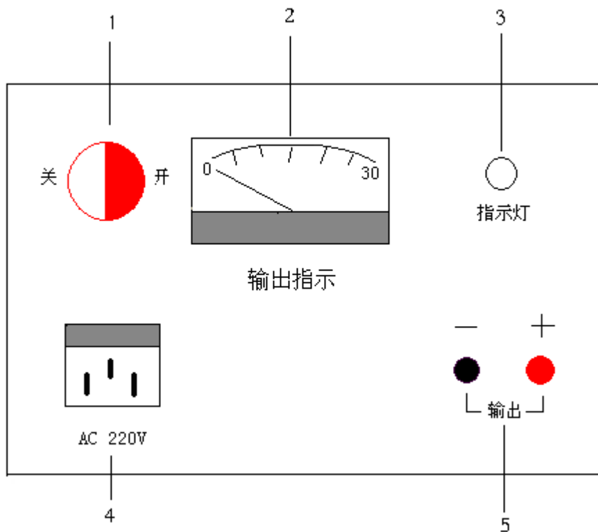
图 3-1 识别仪发射机面板图
