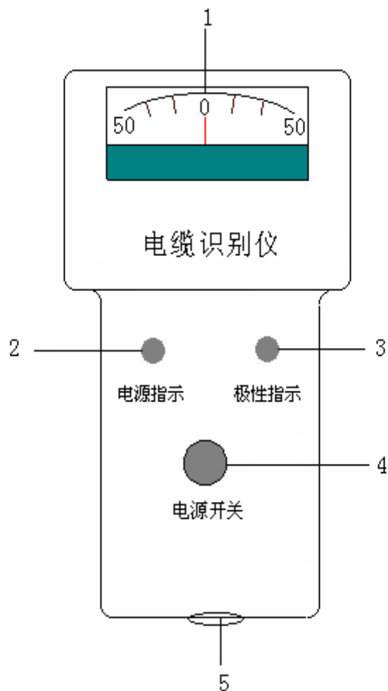
图 3-2 电缆识别仪接收机面板图
