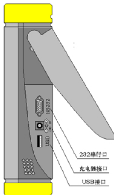
图二、仪器侧面图
