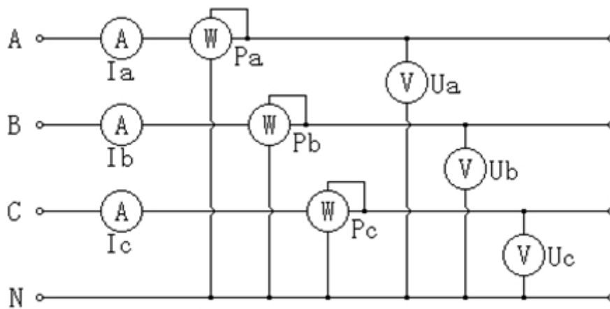
图十八、三相四线计量原理图
