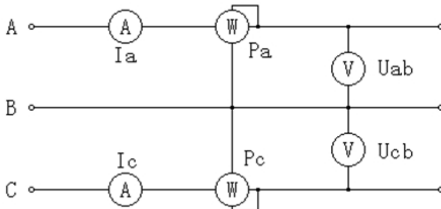
图十七、三相三线计量原理图
